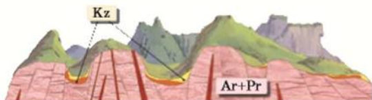
3.3.15. Рельеф и геологическое строение Гвианского плоскогорья
