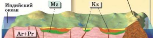
3.4.1. Рельеф и геологическое строение по 30° ю.ш.
