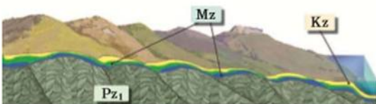
3.3.18. Рельеф и геологическое строение Патагонии
