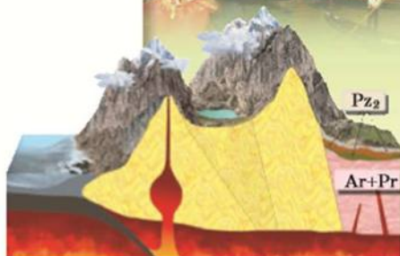
3.3.21. Поперечный разрез центральной части Анд
