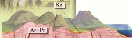
3.3.12. Рельеф и геологическое строение Бразильского плоскогорья
